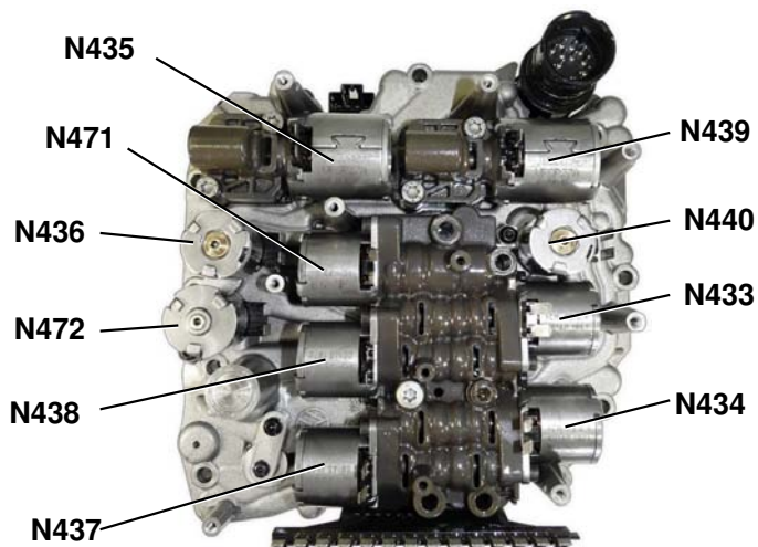
Клапанный блок
